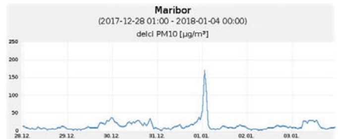
Slika 1: Prikaz vsebnosti delcev PM10 v zraku od 28. 12 2017 do 4. 1. 2018 - vrh prikazuje uporabo pirotehničnih sredstev ob koncu leta 2017
